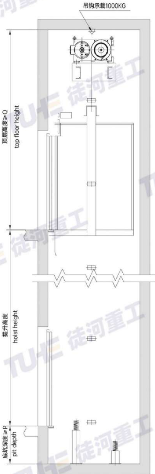
井道立面布置图 Hoistway elevation 1:40
