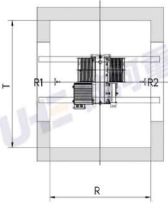
顶层平面图 Top floor plain
