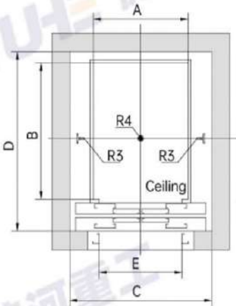
顶层平面图 Top floor plain
